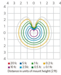
FG 9LED ISOFOOTCANDLE PLOT
